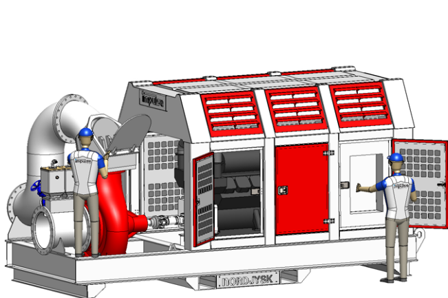
Midlertidig overpumpningsopgave i Aalborg. 4100 m 3 /h x 10 mVs.
